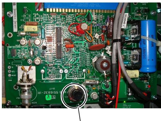
Potentiometer R71
