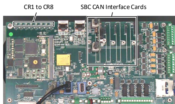
Fig. 5.3. SBC LEDs
