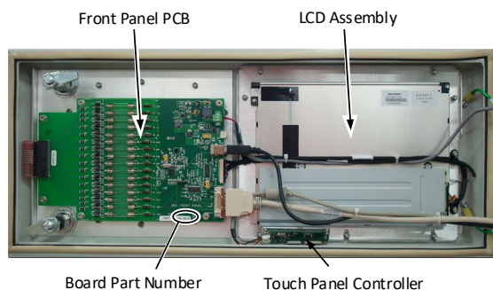
Fig. 8.5. Back of Door
