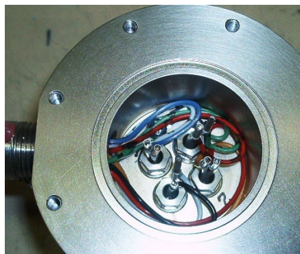
Fig. 8.12. Multiport TCD
