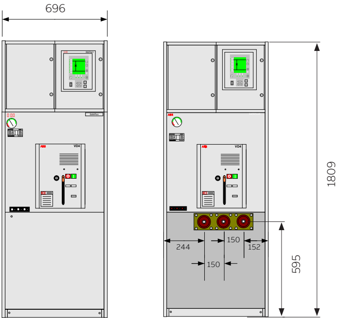
CB modul
