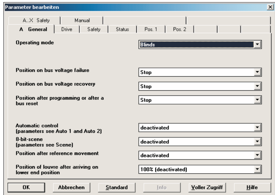
Diagram 28: “A-General” parameter window
