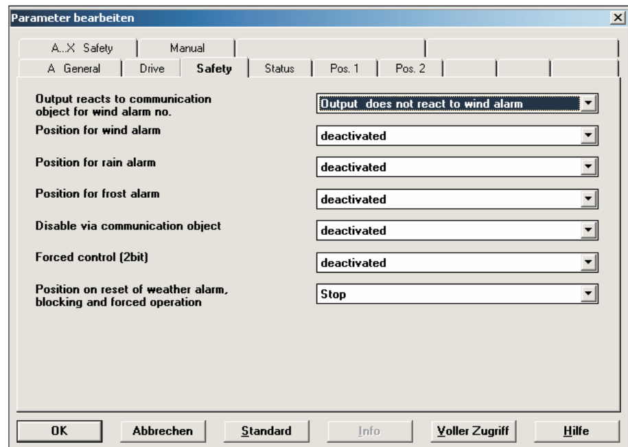
Diagram 30: “Safety” parameter window
