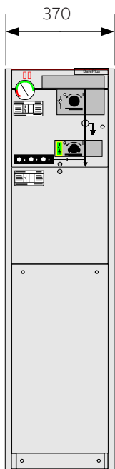
1-way (C-module)
